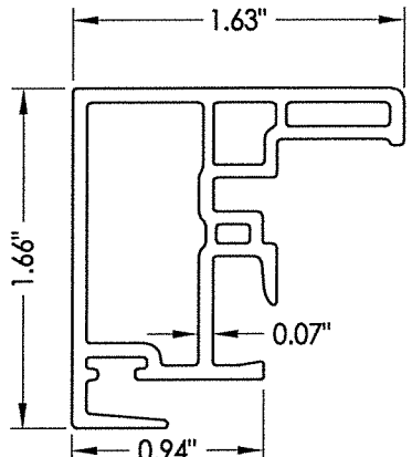
7 LOCK STILE
