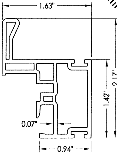
8 HANDLE STILE
